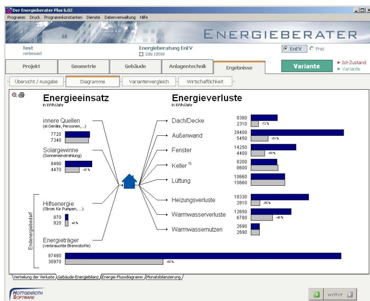
Energiebilanz zur Schwachstellenanalyse im Energieberater von Hottgenroth Software
