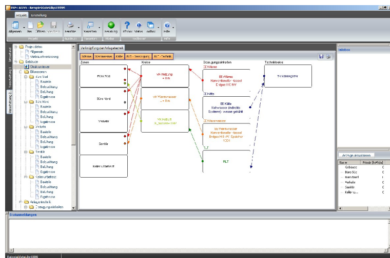
Viewer zur Darstellung der Verknüpfungen von Zonen und Anlagentechnik in 5S:Energy von 5S AG
