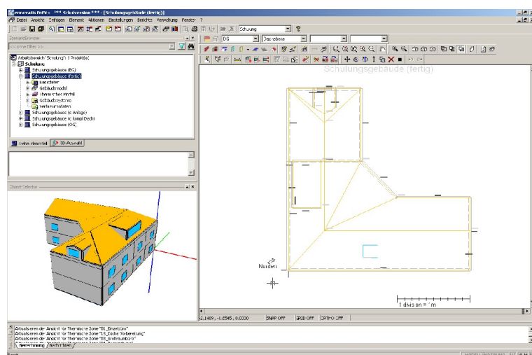
Eingabe eines dreidimensionalen Gebäudemodells in ennovatis EnEV+ von ennovatis GmbH
